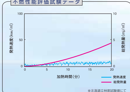
不燃性能評価試験データ
